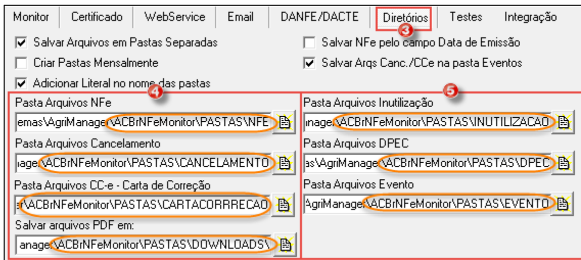
Figura 4- Tela da Configuração do Sistema ACBrNFeMonitor na aba Diretórios.
