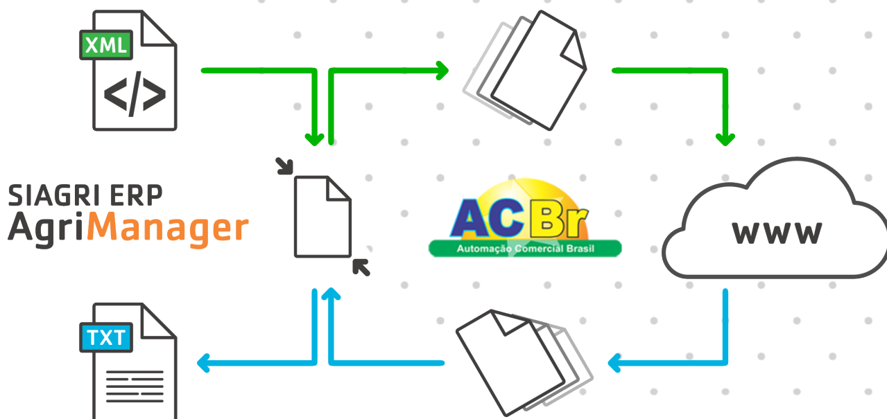
Figura 1 – Ilustração demonstrando o processo entre o SIAGRI AgriManager e o ACBr NFeMonitor.
